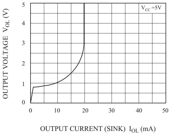
V_{OL} - I_{OL}
