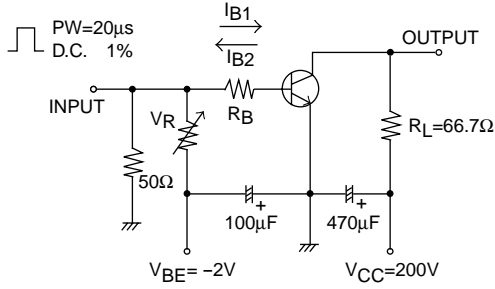
スイッチングタイム測定回路図
